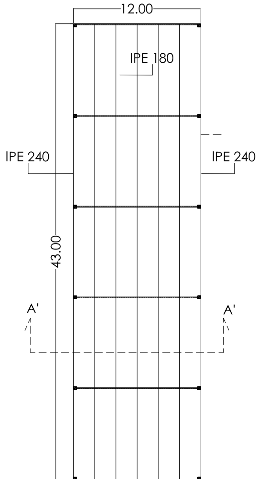
SCHEMA STRUTTURA
